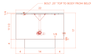
RIGHT ELEVATION
